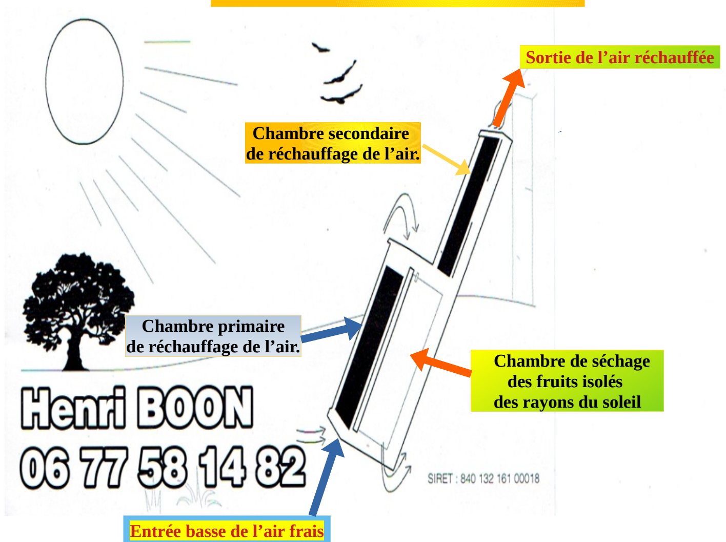
Schéma du principe de circulation de l'air chaud pour le séchage.
